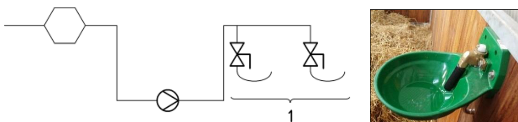
Figur 6.5. Hvis drikkebrugene (1) er med indbygget luftgab, er det ikke nødvendigt med ekstra sikring. Hvis der ikke er luftgab i trugene, skal der monteres en kategori 5 sikring på ledningen til disse.
