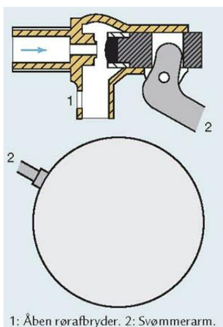
1: Åben rørafbryder. 2: Svømmerarm.
