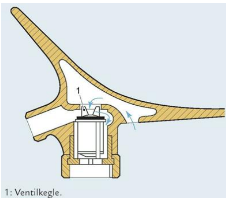
1: Ventilkegle.
